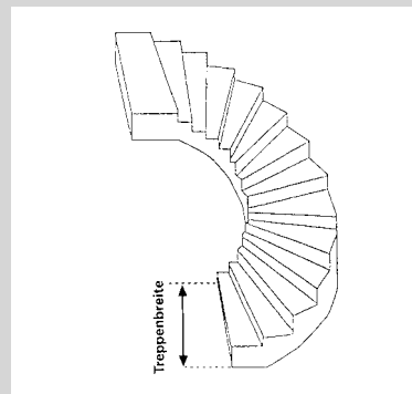
4. Wendeltreppe 180° gebogen
